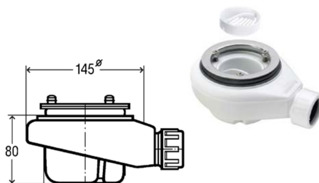
Detalle válvula Viega Tempoplex 80
