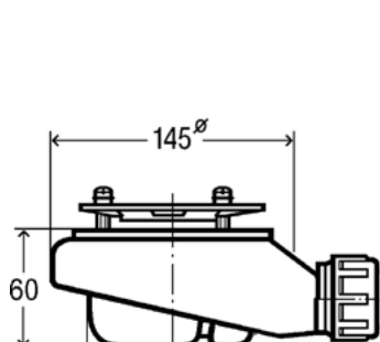
Detalle válvula Viega Tempoplex 60
