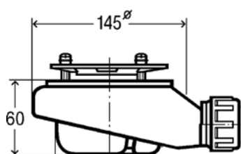
Detalle válvula Viega Tempoplex 60
