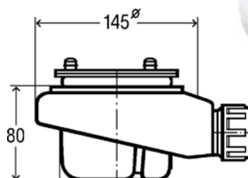
Detalle válvula Viega Tempoplex 80
