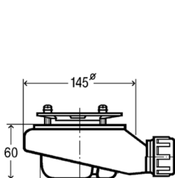
Detalle válvula Viega Tempoplex 60
