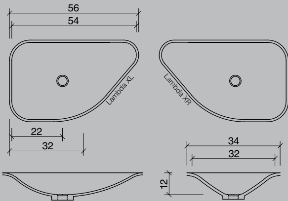
Lambda XL : Válvula a la izquierda Lambda XR : Válvula a la derecha
